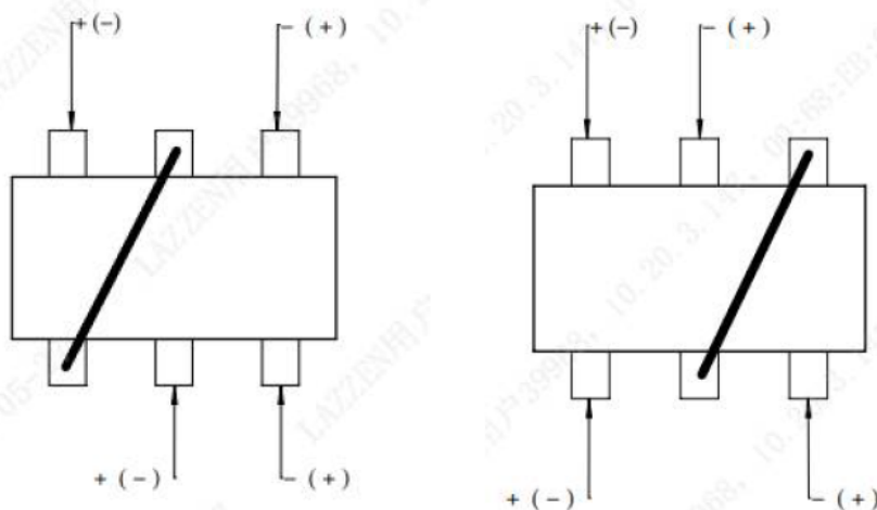
3P 接线图
